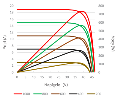
Charakterystyka prądowo – napięciowa (700W)
